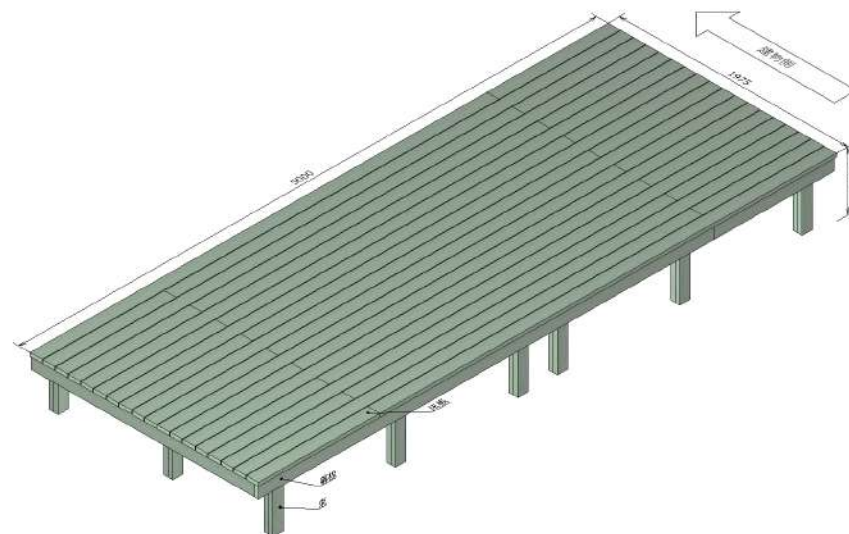
等角図(左)
