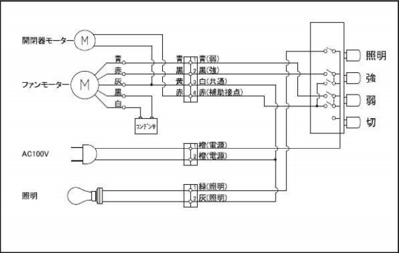
□結線図
